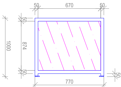
ELEVATION BB
